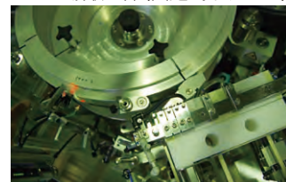
ラベル自動修正装置
