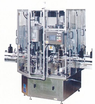
CLS-020P型P.P.キャッパー P.P. capper 2 Head
